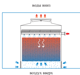
Противоток Конфигурация
