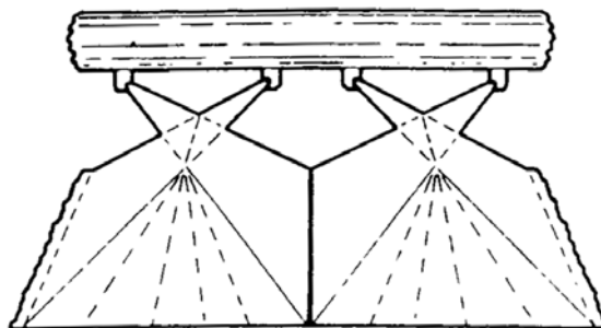
Рисунок 6: Структура разбрызгивания форсунок для градиент испарительного типа
