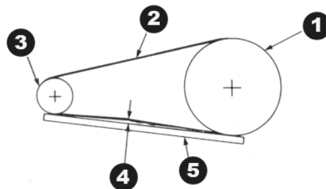
Рисунок 3: Регулировка ремня вентилятора
