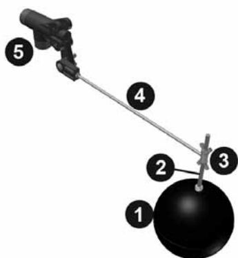
Рисунок 2: Узел клапана подпитки водой
